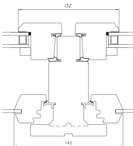
Pystyjakokarmi
