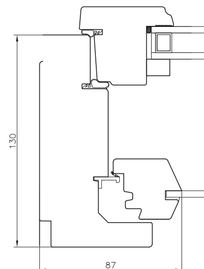
Sivukarmi
