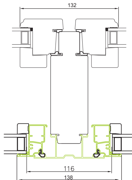
Pystyjakokarmi
